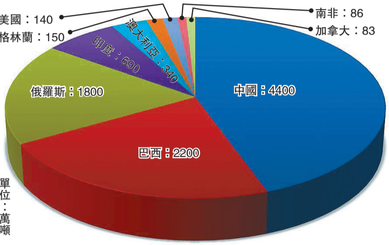
截至2018年，全球稀土資源分布
